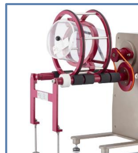
Mélangeur tambour
